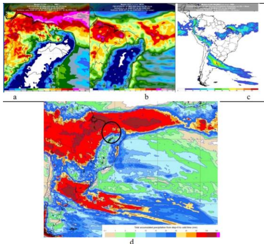
Figura 1- Acumulado de chuva entre os dias 24/02 e 02/03/2025 de acordo com os modelos numéricos de previsão do tempo Cosmo (a), GFS (b) e ECMWF (d) e probabilidade de chuva acima de 20 mm para as próximas 132 horas (até 01/03) pelo modelo ICON (c). Vale destacar que, as imagens são meramente ilustrativas e refletem apenas uma das muitas variáveis meteorológicas utilizadas na elaboração das previsões de tempo.
